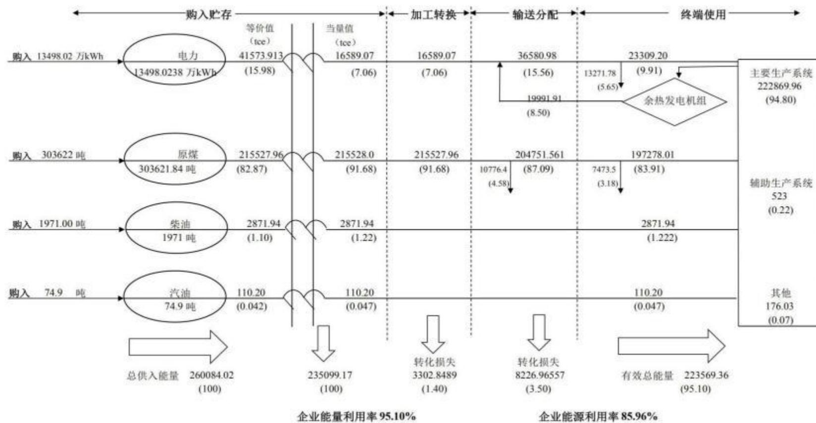
图 1 企业能量平衡图
